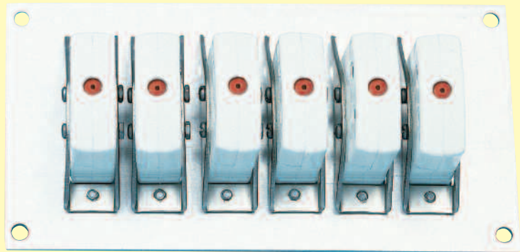
MTCコネクター用パネル取付ブラケット:型式MTACL パネル 開口: 23.72 H x 8.08 mm W (0.93 x 0.32")
