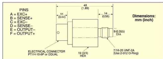
公称寸法図: 単位 mm (インチ)
